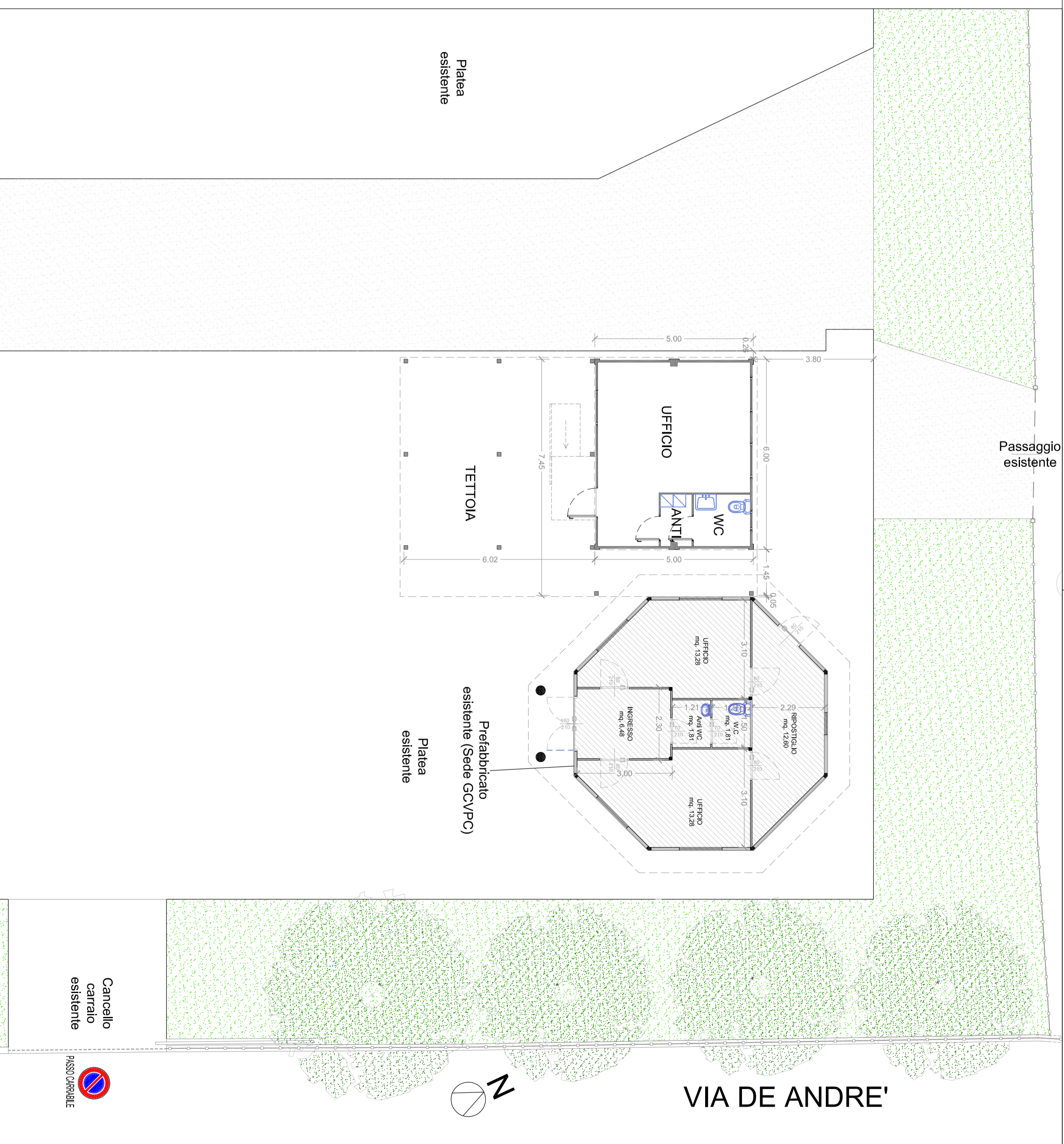
PLANIMETRIA SISTEMAZIONE ESTERNA E POSIZIONAMENTO PREFABBRICATI 1:100
